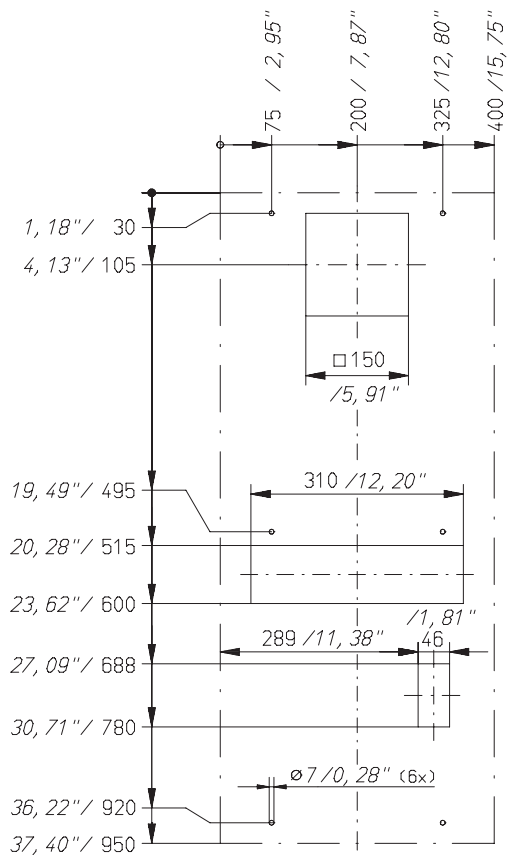
Lochbild Schrankanbau
